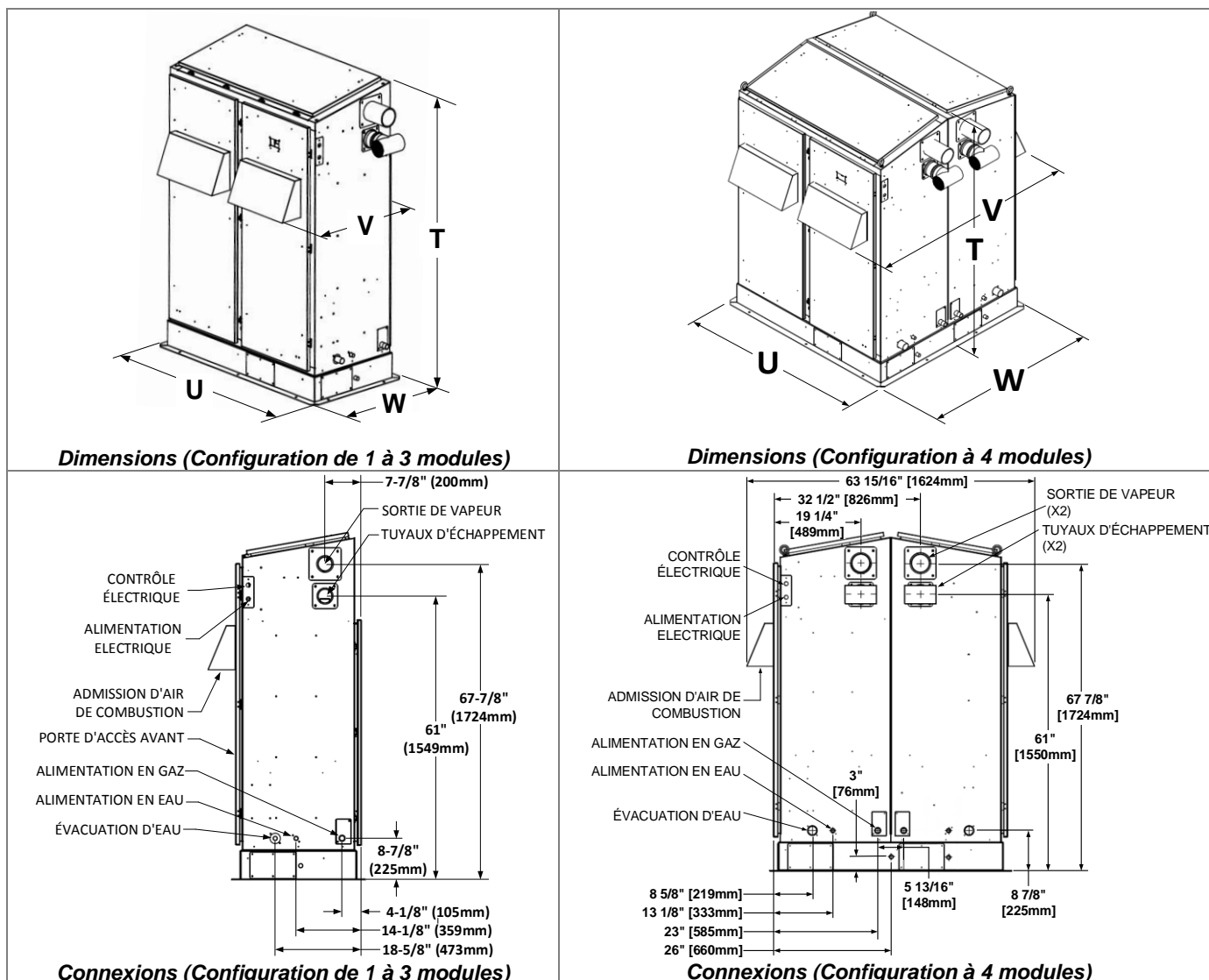
Illustration 6 - Boîtier extérieur
