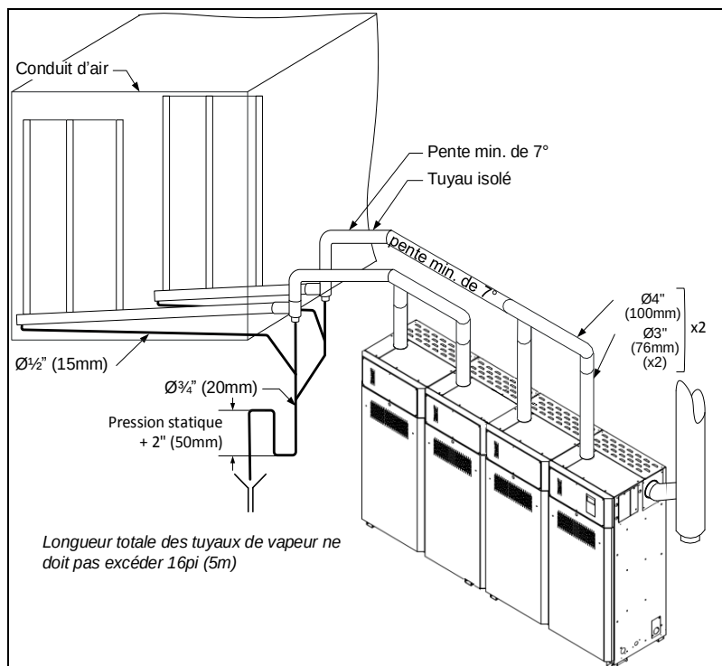
Illustration 26 - Tuyaux de vapeur Multi-Steam (SKG4-N7104 à 8104)
