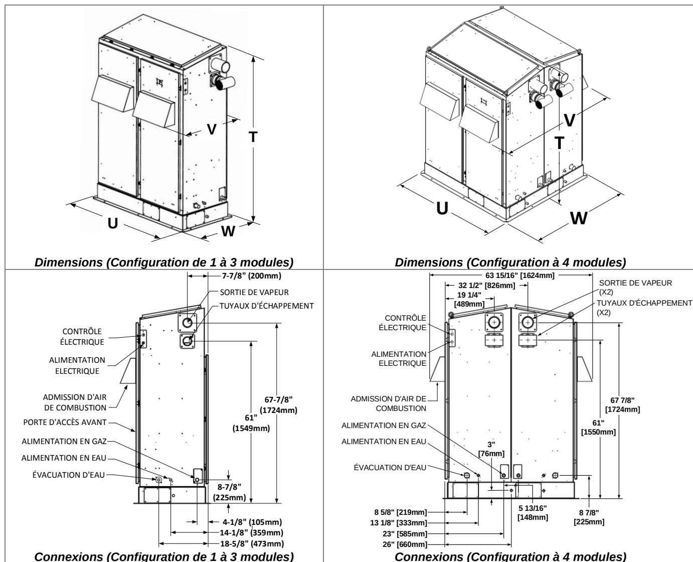
Illustration 6 - Boîtier extérieur
