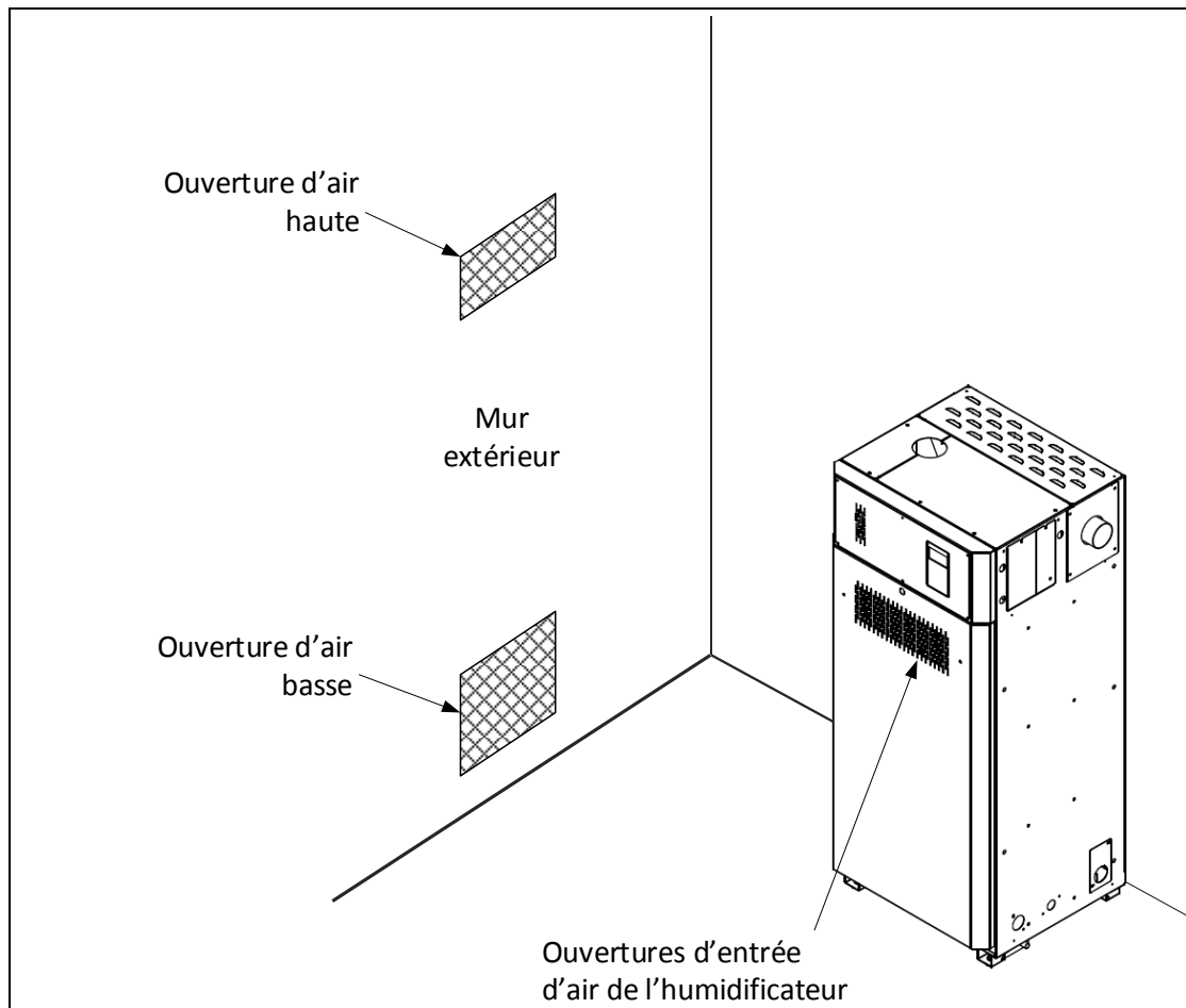
Illustration 33 - Configuration de la ventilation naturelle
