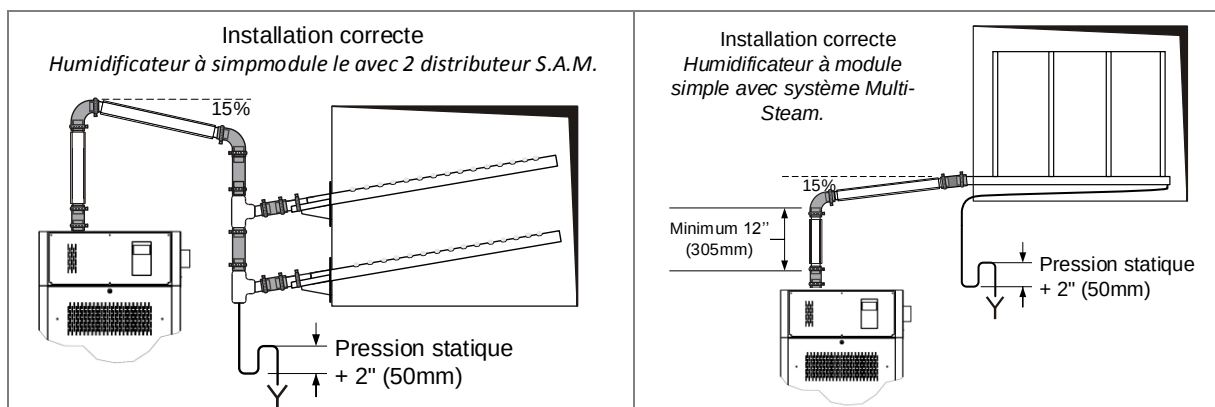
Illustration 14 - Tuyaux de distribution de vapeur : bonne installation
