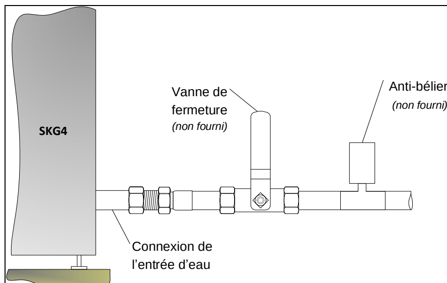
Illustration 28 - Connexion d'alimentation d'eau
