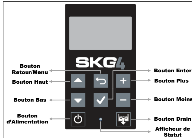
Illustration 48 - Contrôleur SKG4
