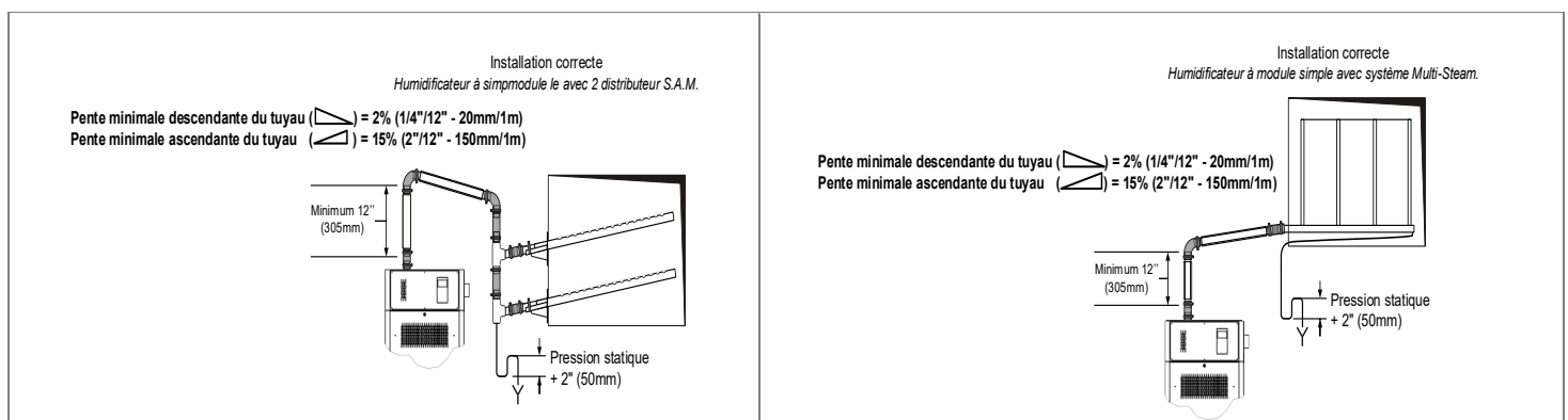
Illustration 14 - Tuyaux de distribution de vapeur : bonne installation
