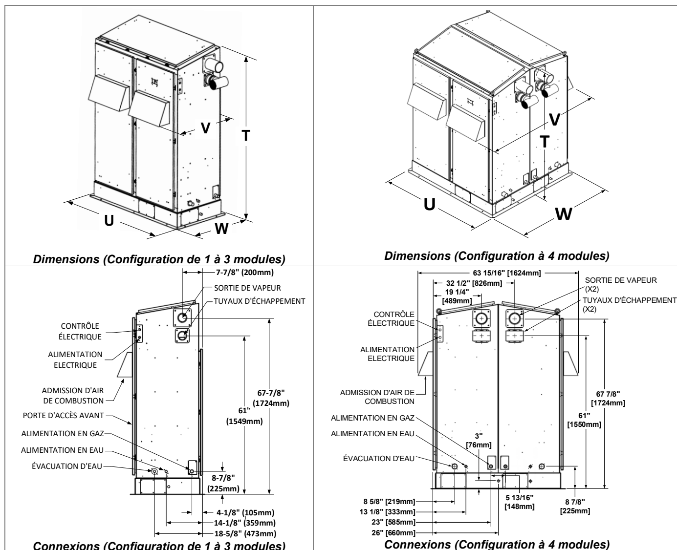
Illustration 6 - Boîtier extérieur
