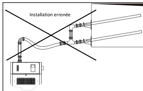
Illustration 13 - Tuyaux de distribution de vapeur : installation erronée
