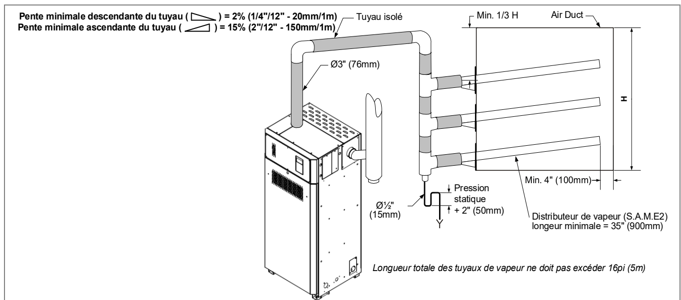
Illustration 20 - Tuyaux de vapeur S.A.M.E2 (SKG4-N1551 à 2101)
