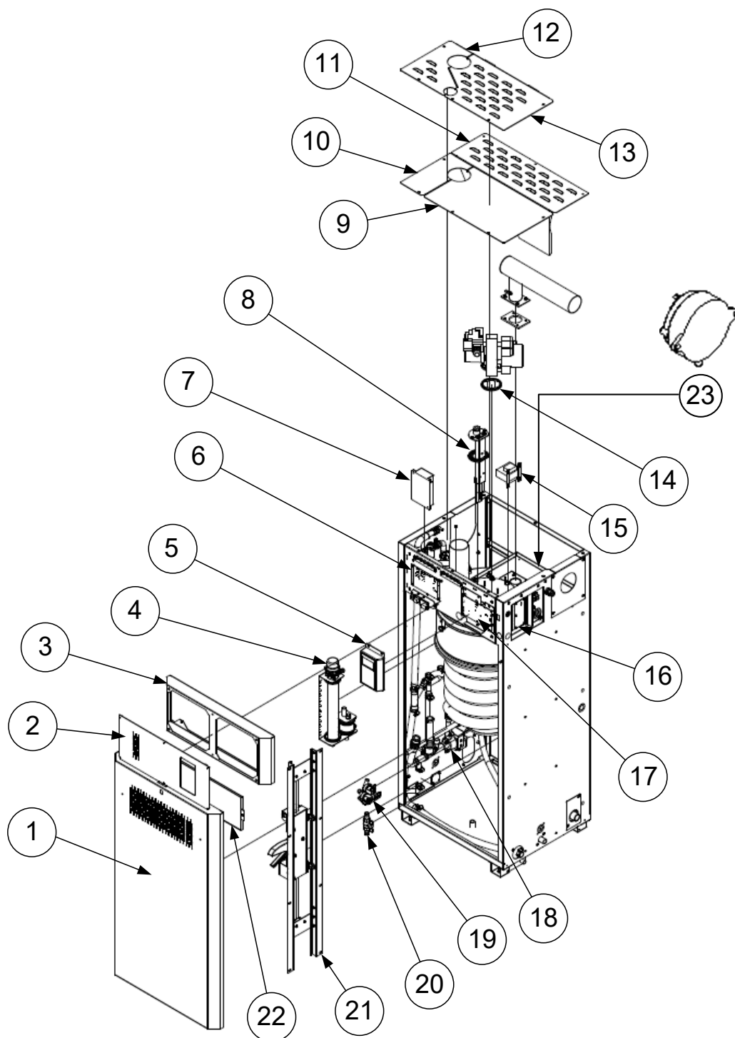
Illustration 52 - Vue explosée générale
