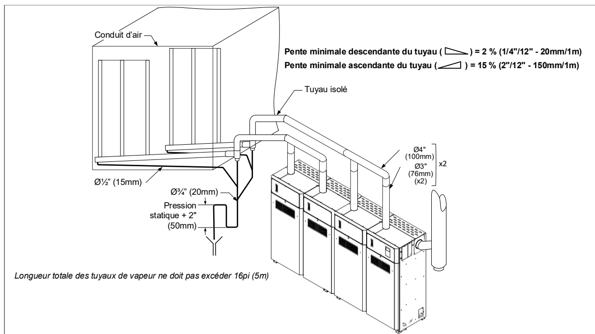
Illustration 26 - Tuyaux de vapeur Multi-Steam (SKG4-N7104 à 8104)
