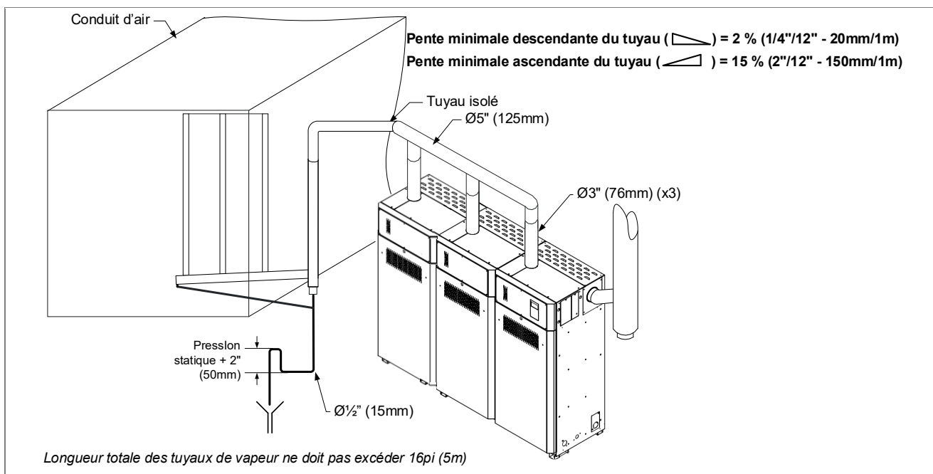
Illustration 25 - Tuyaux de vapeur Multi-Steam (SKG4-N5053 à 6103)
