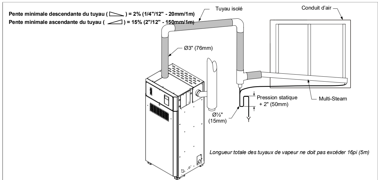
Illustration 23 - Tuyaux de vapeur Multi-Steam (SKG4-N1101 à 2651)
