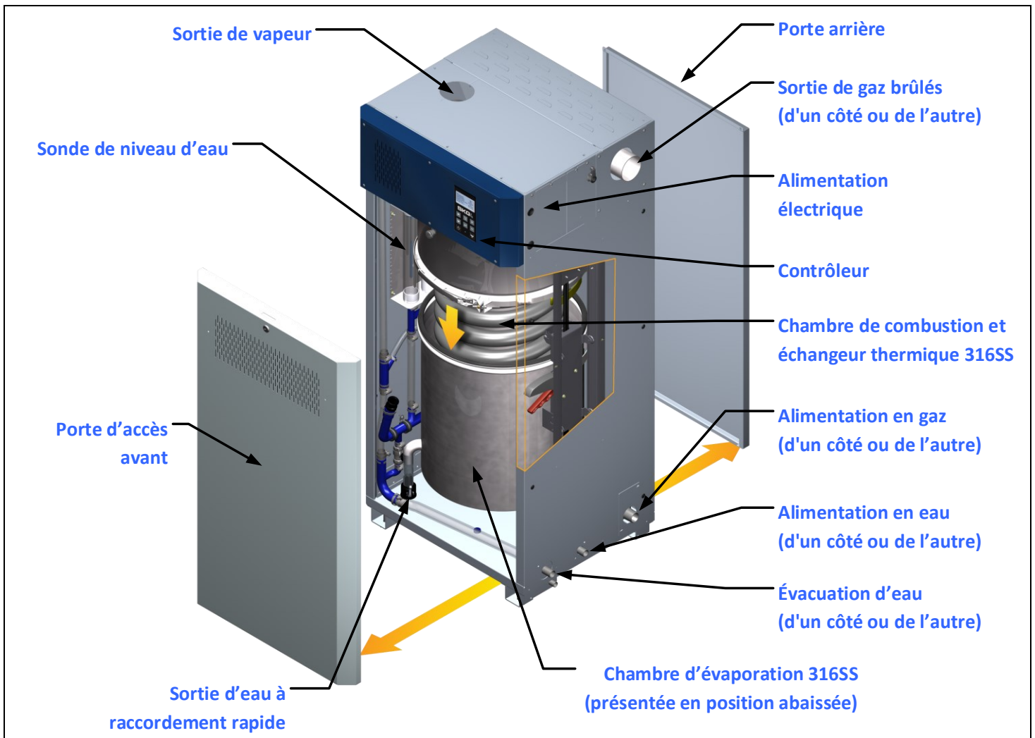
Illustration 2 - Aperçu de l'humidificateur
