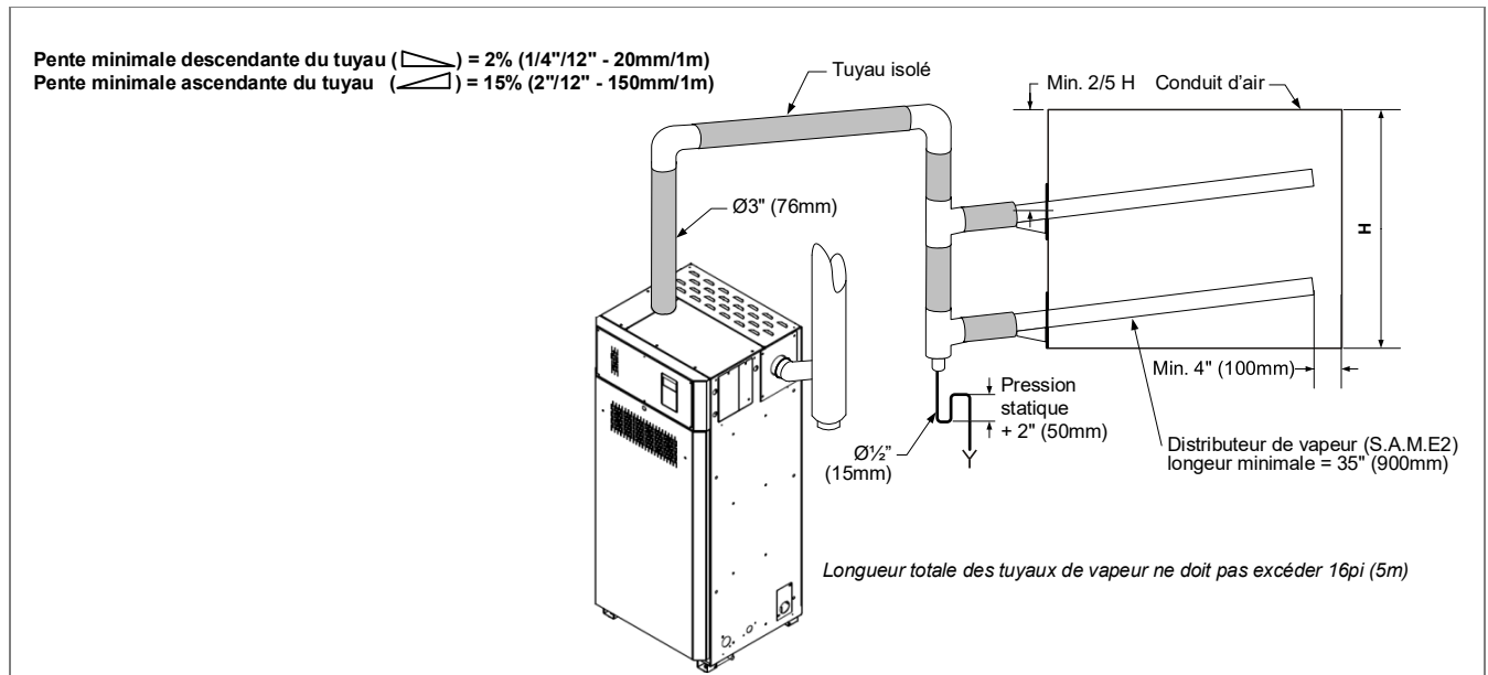
Illustration 19 - Tuyaux de vapeur S.A.M.E2 (SKG4-N1101)
