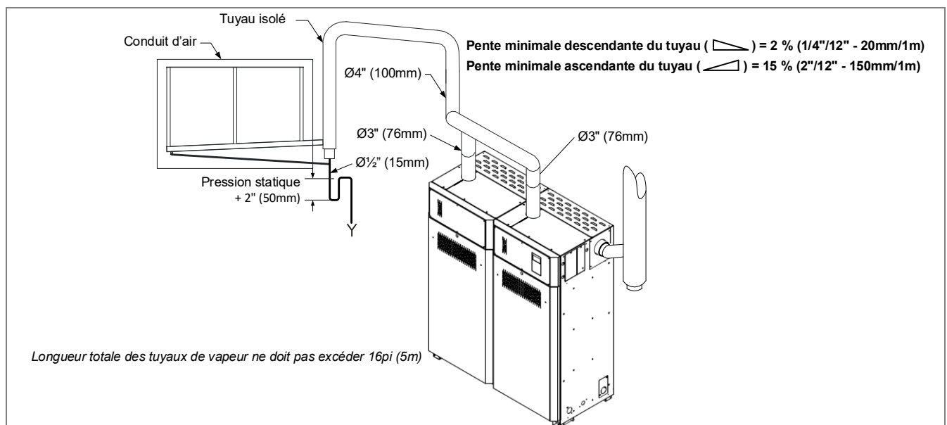
Illustration 24 - Tuyaux de vapeur Multi-Steam (SKG4-N2652 à 4052)
