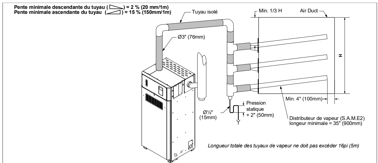
Illustration 20 - Tuyaux de vapeur S.A.M.E2 (SKG4-E0701 à 1001)
