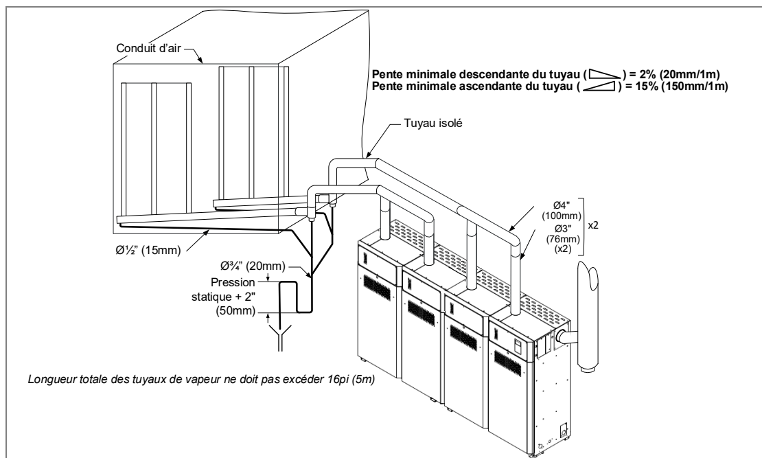
Illustration 26 - Tuyaux de vapeur Multi-Steam (SKG4-E3504 à 4004)
