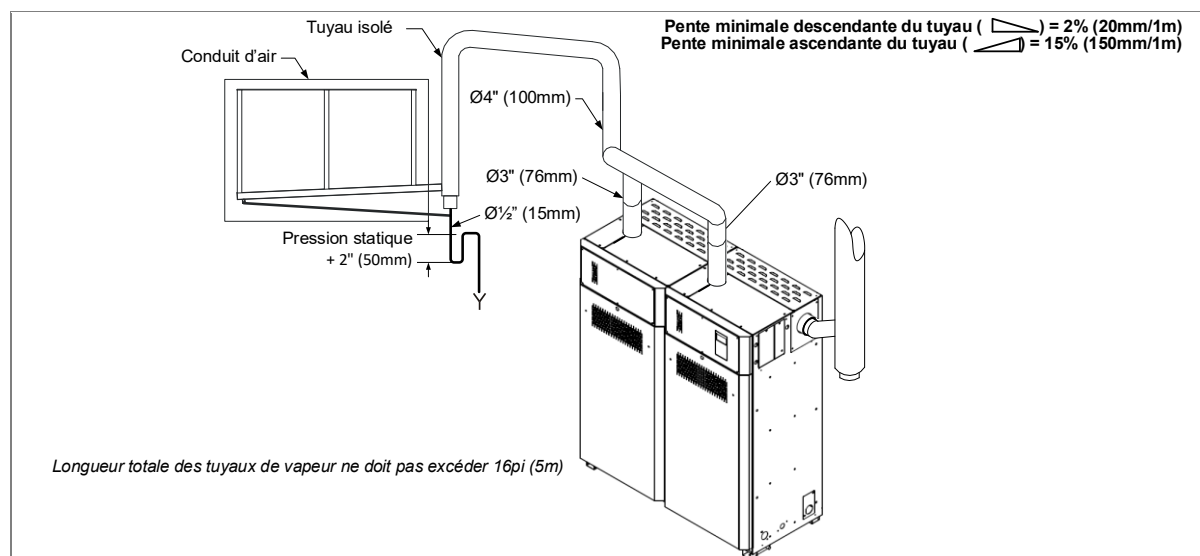
Illustration 24 - Tuyaux de vapeur Multi-Steam (SKG4-E1202 à 2002)
