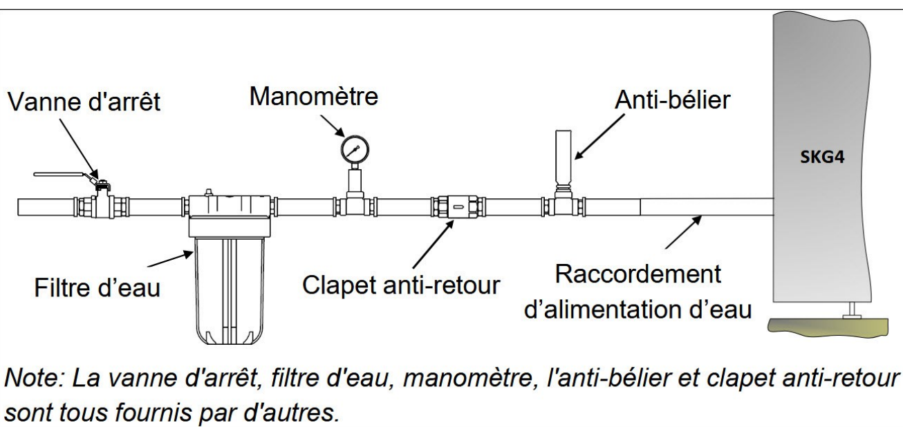
Illustration 28 - Connexion d'alimentation d'eau
