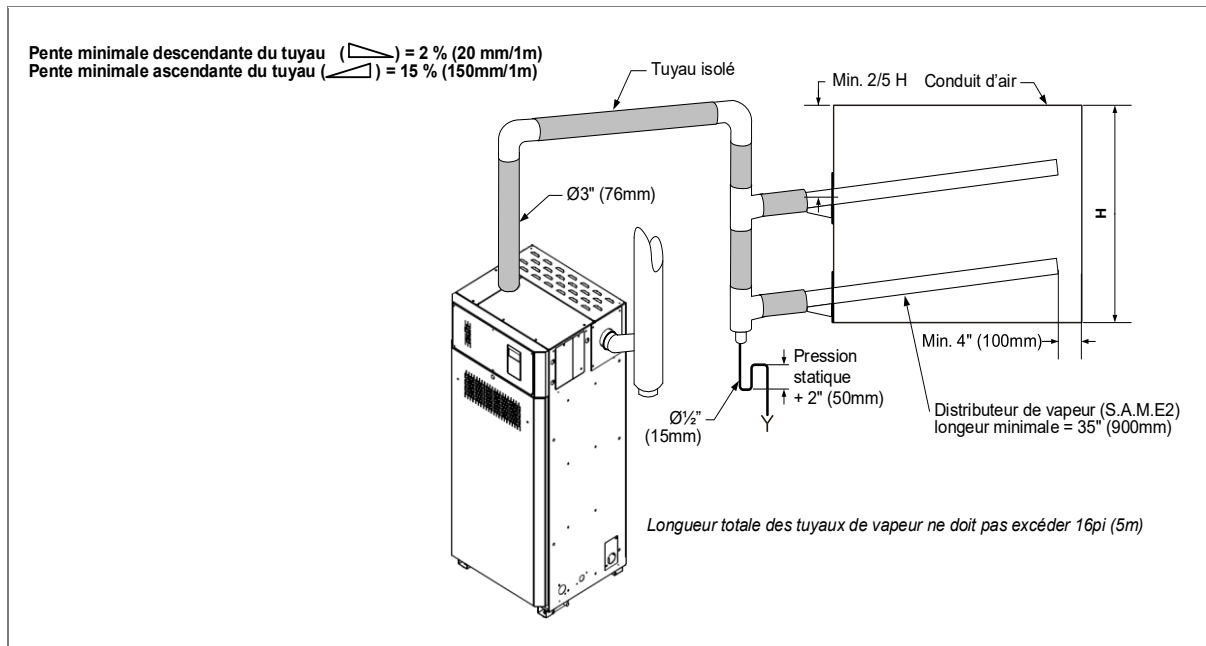
Illustration 19 - Tuyaux de vapeur S.A.M.E2 (SKG4-E0501)
