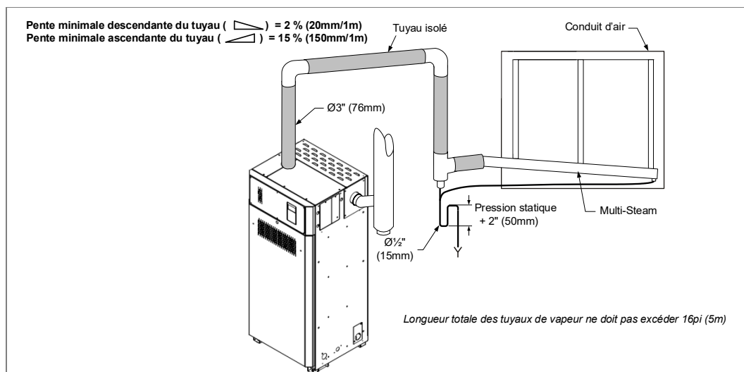
Illustration 23 - Tuyaux de vapeur Multi-Steam (SKG4-E0501 à 1001)
