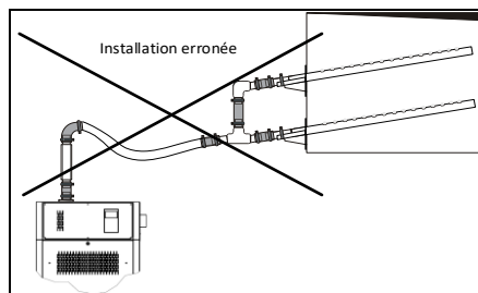
Illustration 13 - Tuyaux de distribution de vapeur : installation erronée
