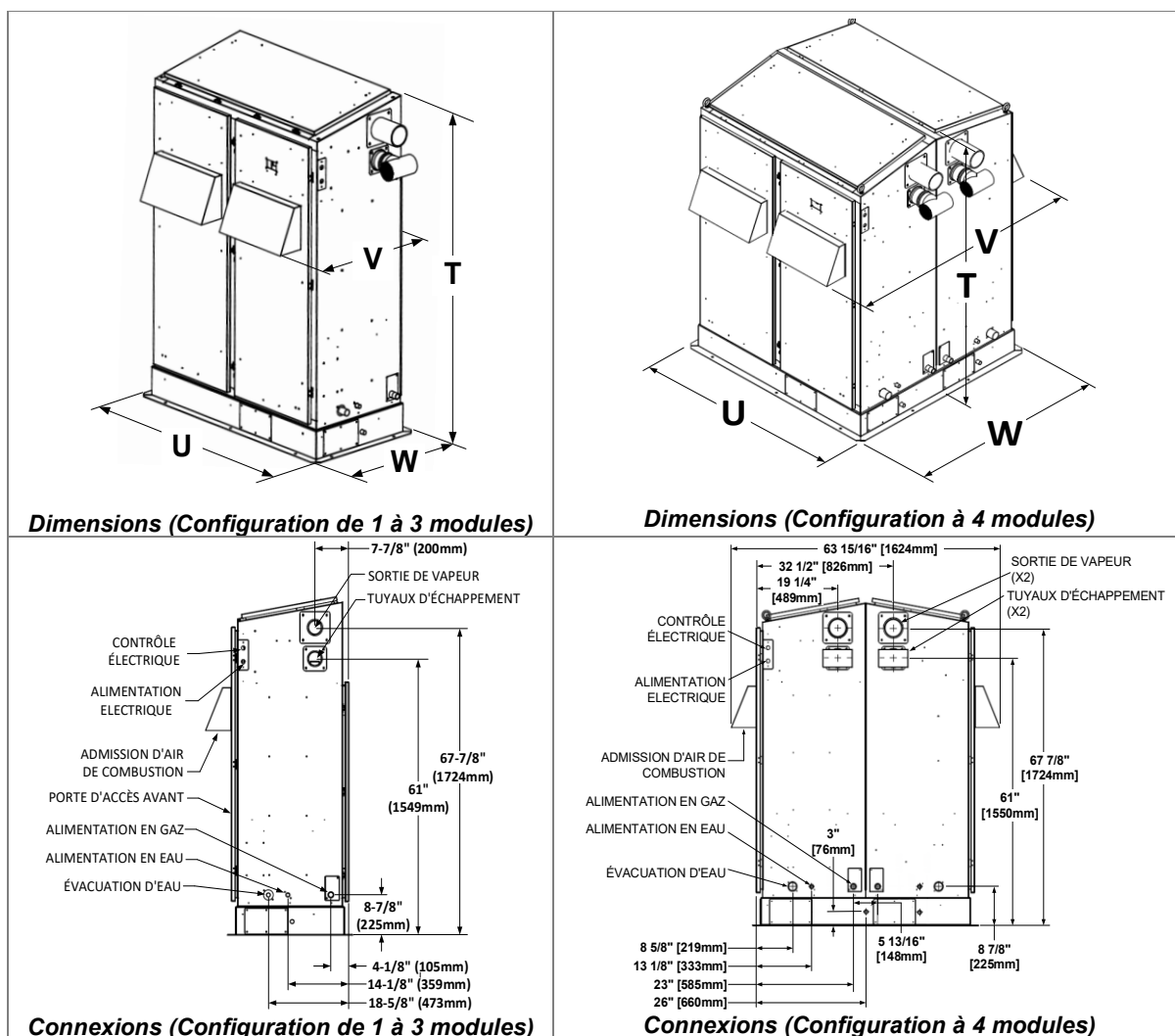
Illustration 6 - Boîtier extérieur
