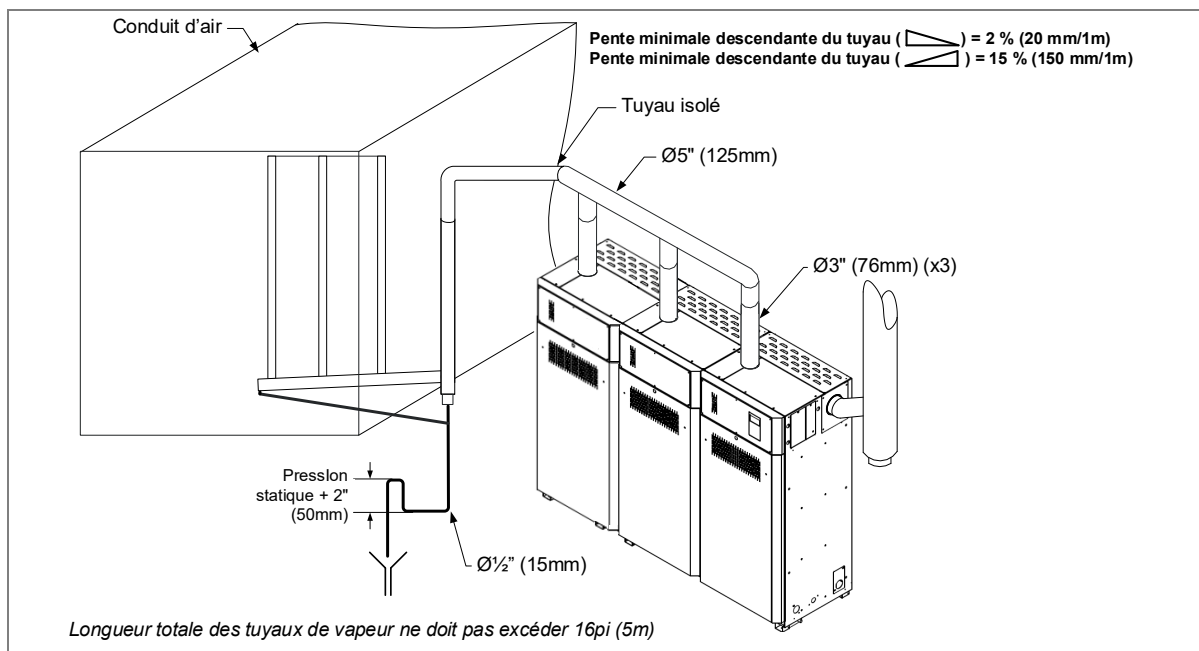
Illustration 25 - Tuyaux de vapeur Multi-Steam (SKG4-E2503 à 3003)
