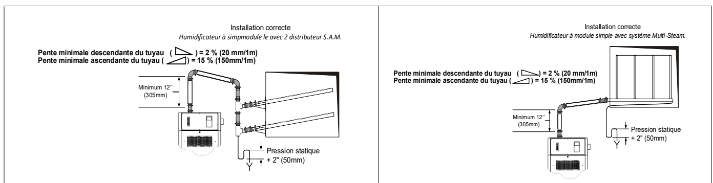
Illustration 14 - Tuyaux de distribution de vapeur : bonne installation
