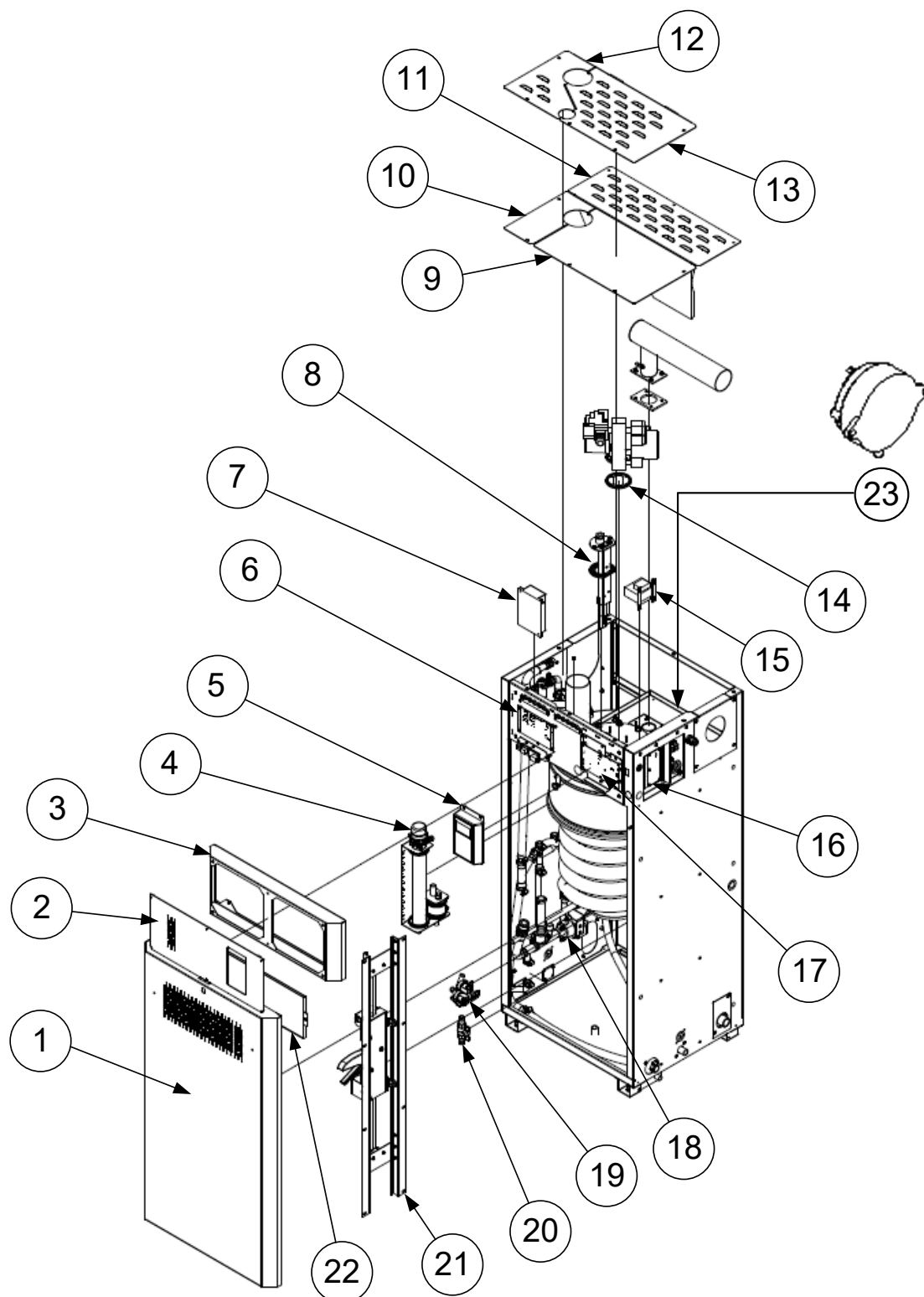
Illustration 52 - Vue explosée générale
