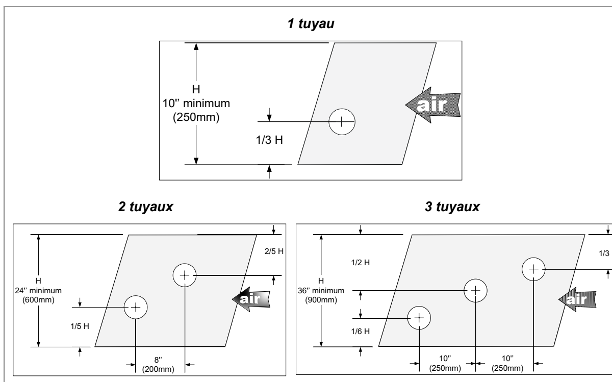
Illustration 22 - Emplacement de tuyaux de 51 mm de diamètre : conduit horizontal
