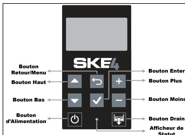
Illustration 42 - Contrôleur SKE4
