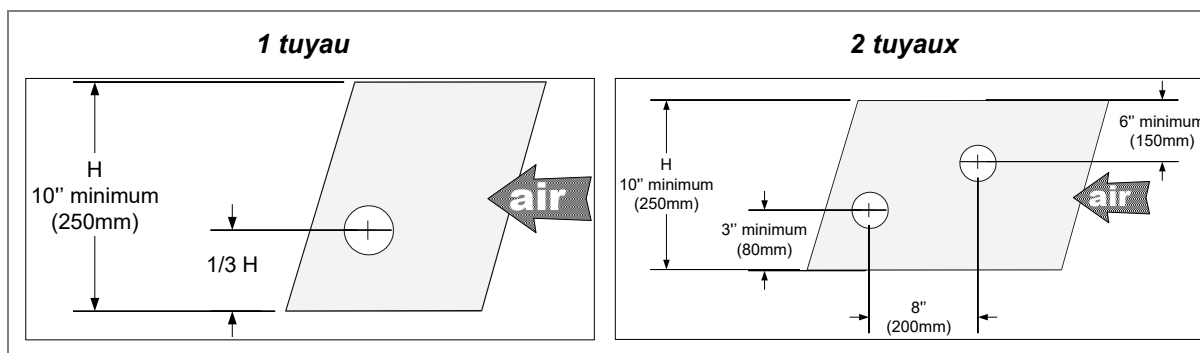
Illustration 21 - Emplacement de tuyaux de 35 mm de diamètre : conduit horizontal
