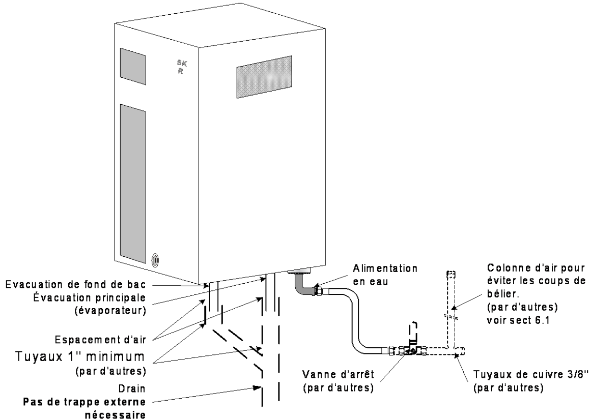
(Illus. 8a) Installation recommandée
