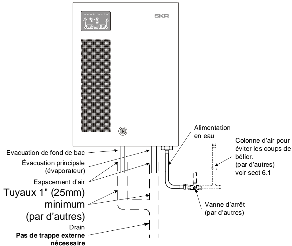
(Illus. 10a) Installation recommandée
