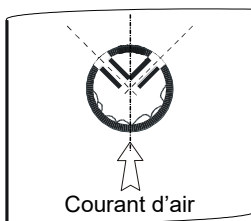
(Illus. 8d) Alignement du distributeur de vapeur dans un conduit vertical pour le SKR-14/25
