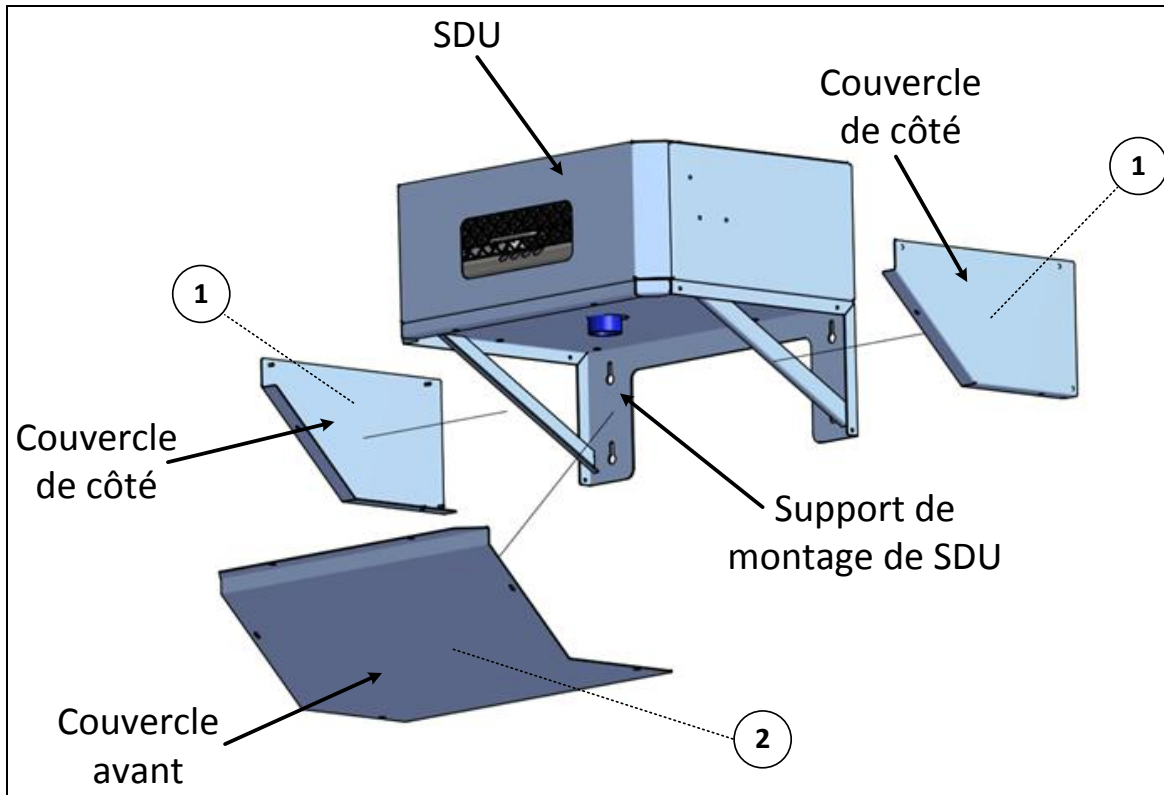
Illustration 34 - Installation du couvercle pour SDU à distance
