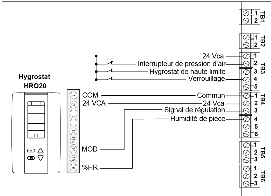
Illustration 46 - Signal de contrôle d'un hygromètre HRO20
