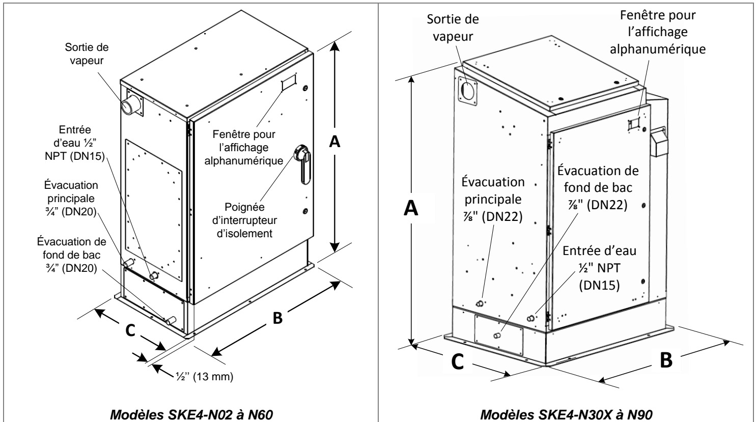
Illustration 5 - Boîtier extérieur
