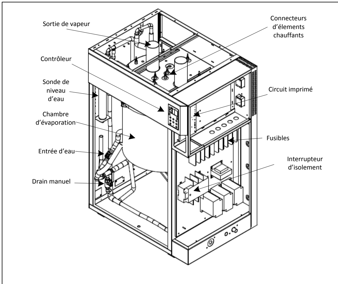
Illustration 2 - Aperçu de l'humidificateur (SKE4-N30X à N90)
