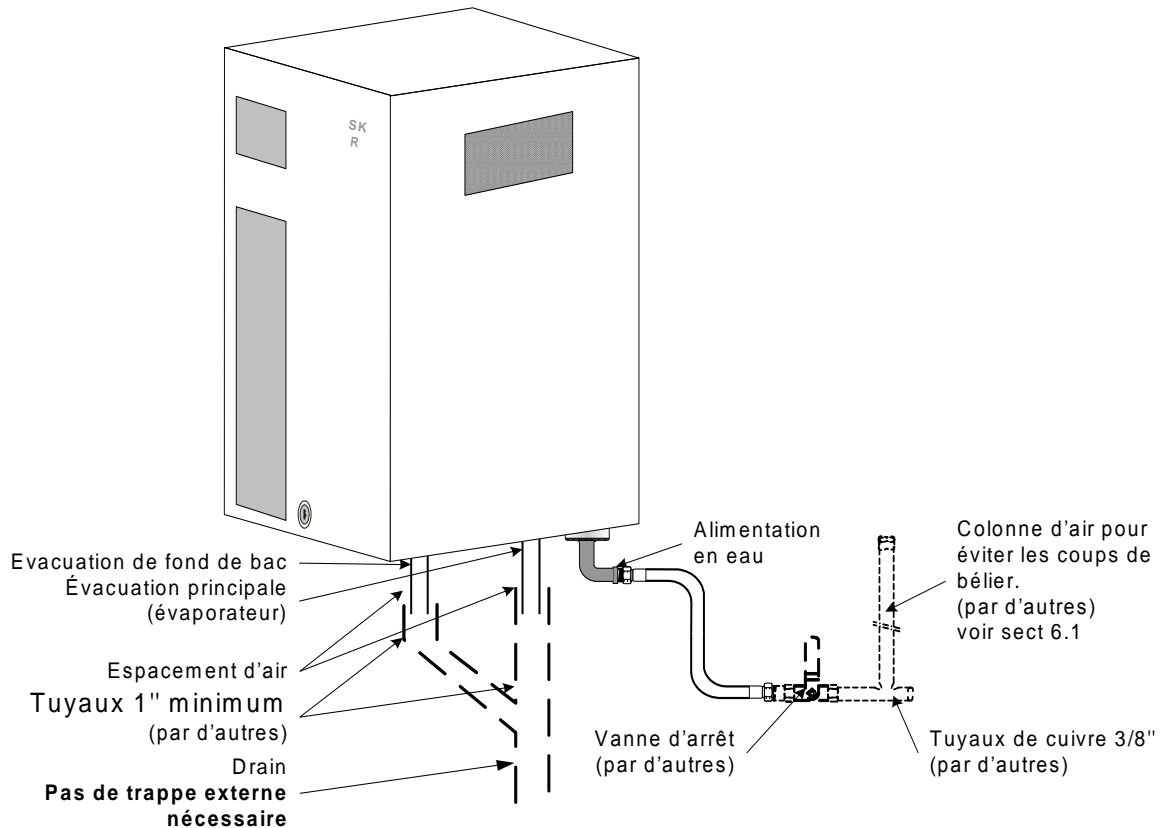
(Illus. 8a) Installation recommandée
