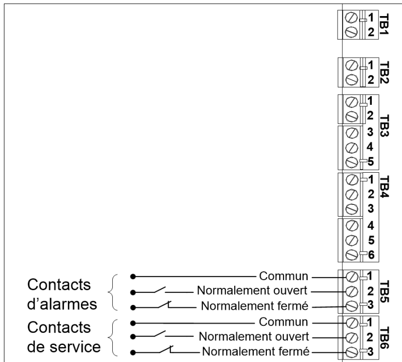
Illustration 38 - Câblage des contacts d'alarmes et de service
