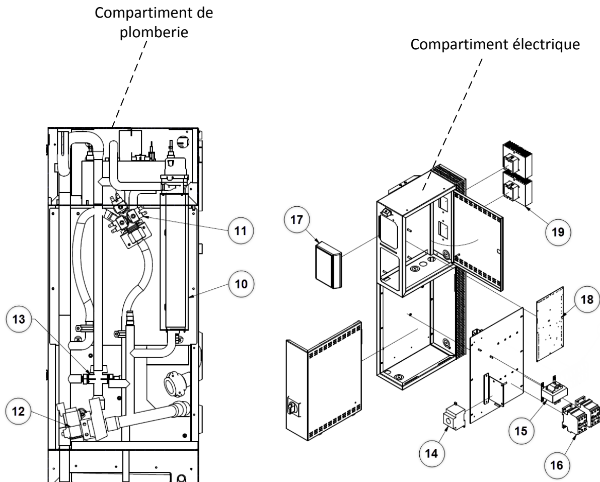
Illustration 51 - Vue explosée partie 2
