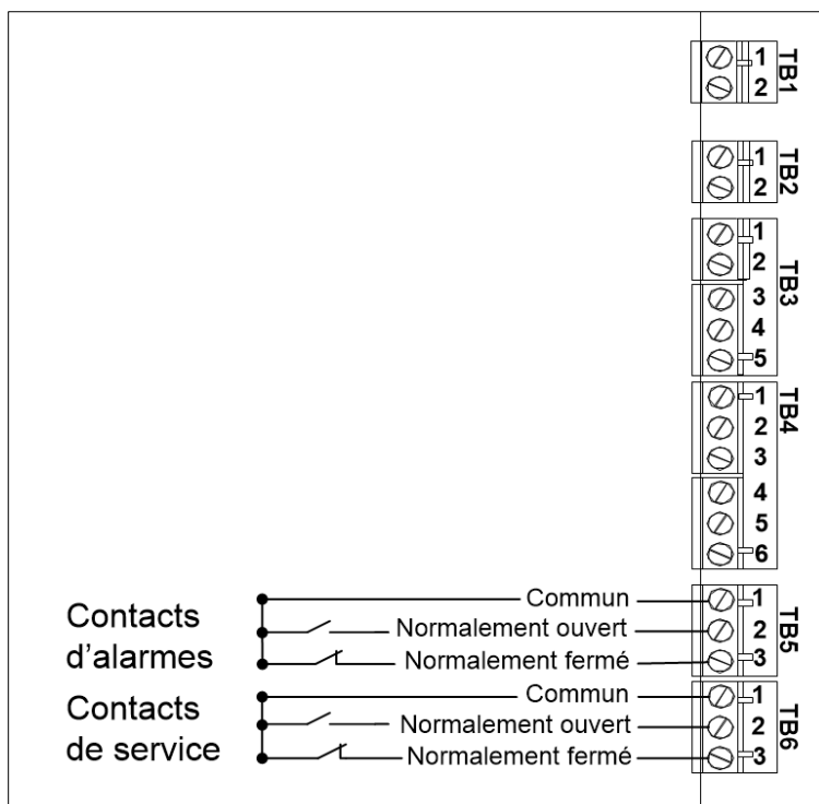
Illustration 38 - Câblage des contacts d'alarmes et de service
