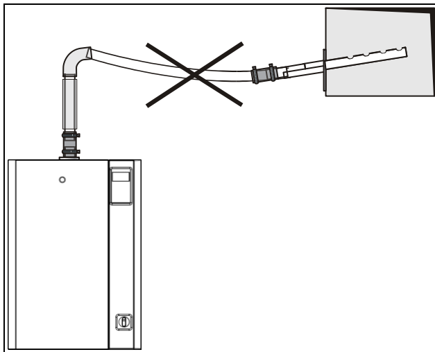
Illustration 24 - Installation erronée de la sortie de vapeur
