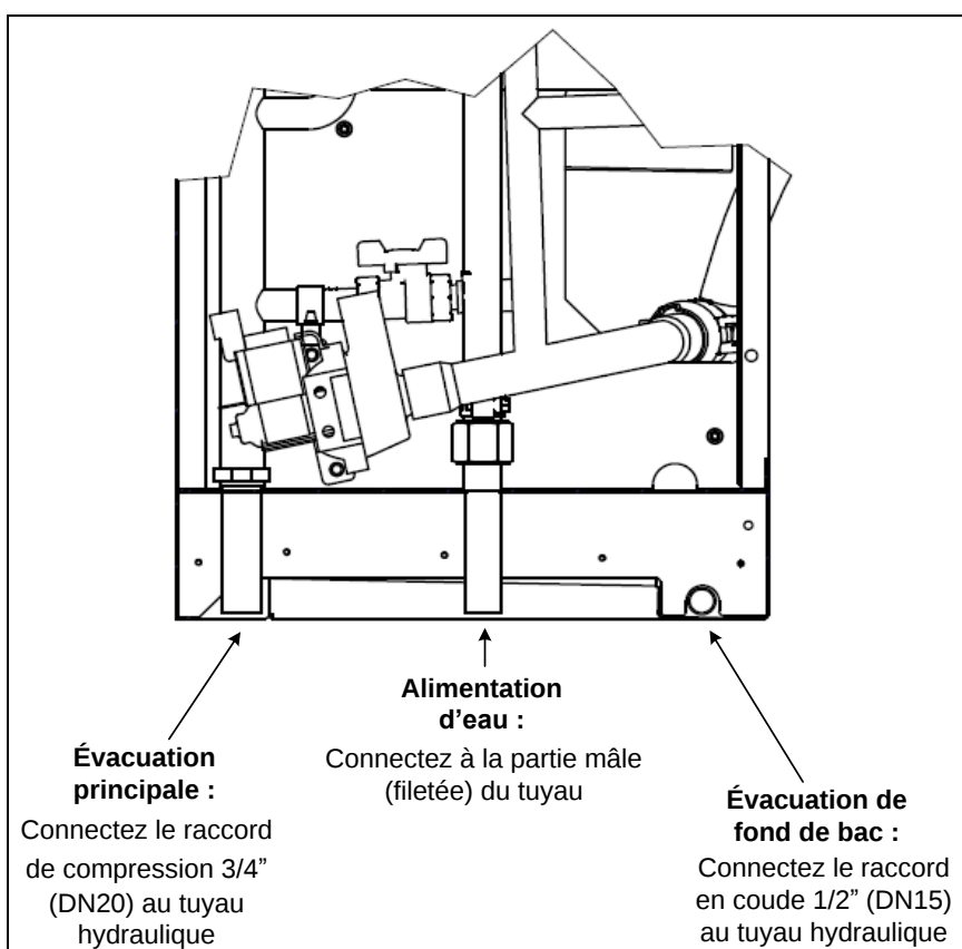
Illustration 31 - Raccordement d'alimentation et d'évacuation d'eau
