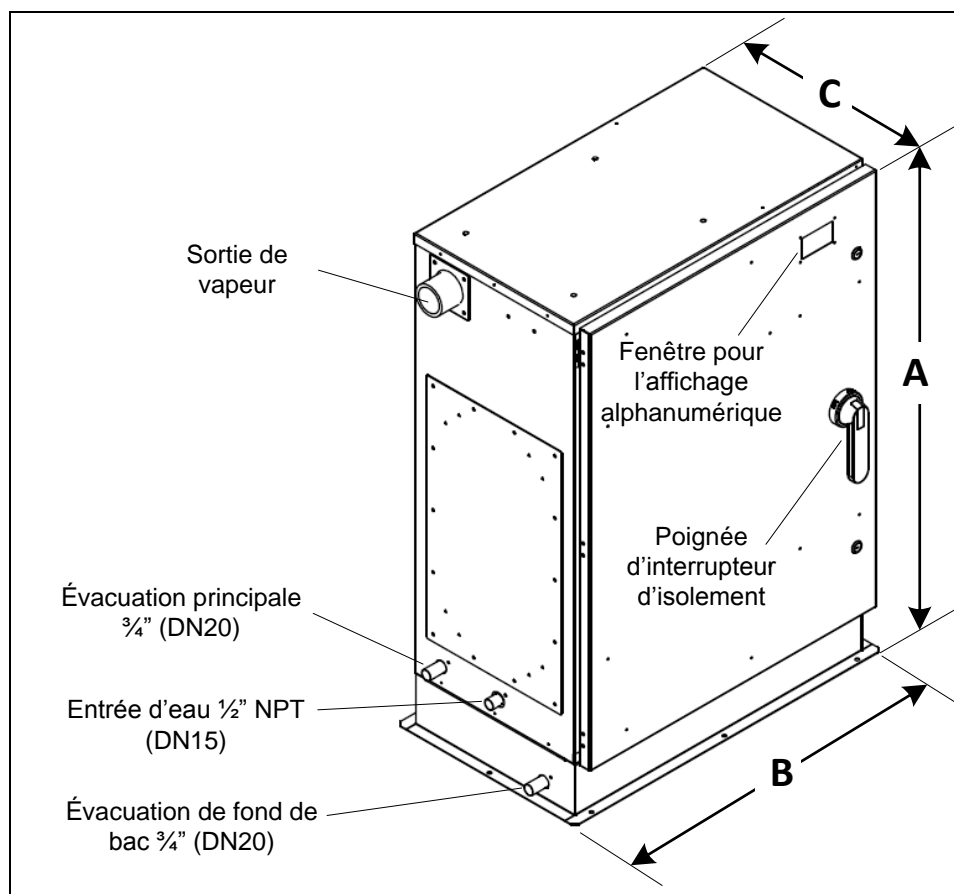
Illustration 6 - Boîtier extérieur (OSP)
