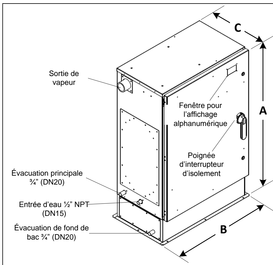
Illustration 5 - Boîtier extérieur
