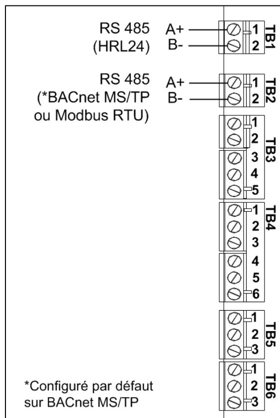
Illustration 49 - Connexions au réseau de communication
