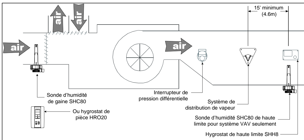
Illustration 50 - Emplacement des contrôles (vapeur distribuée dans un conduit ou CTA)
