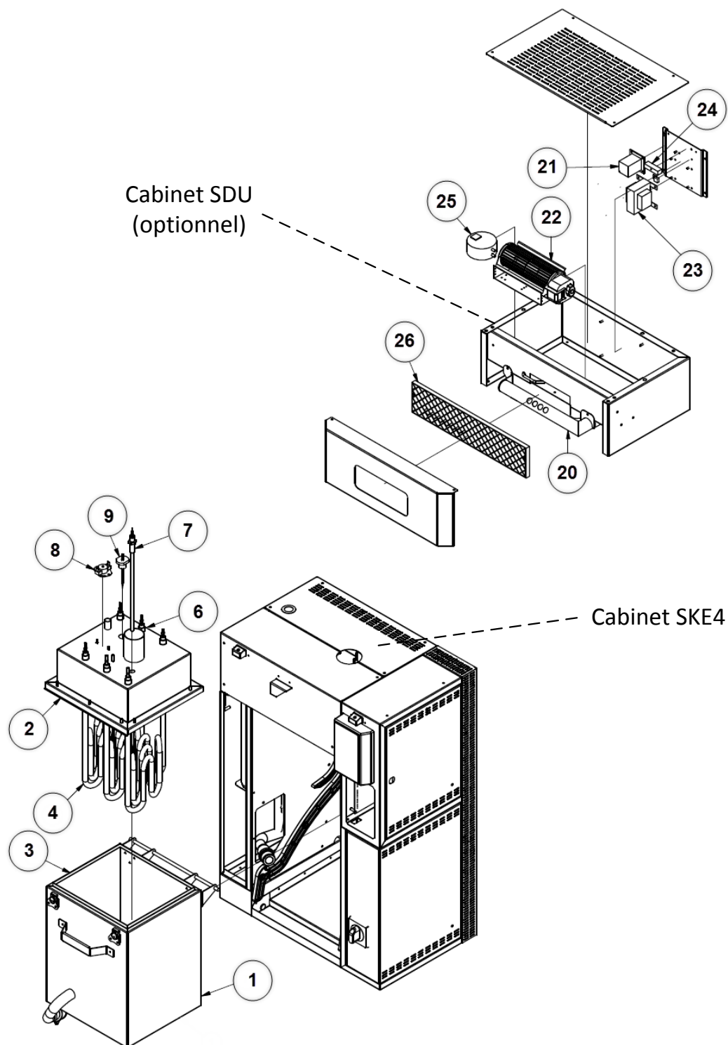
Illustration 55 - Vue explosée partie 1
