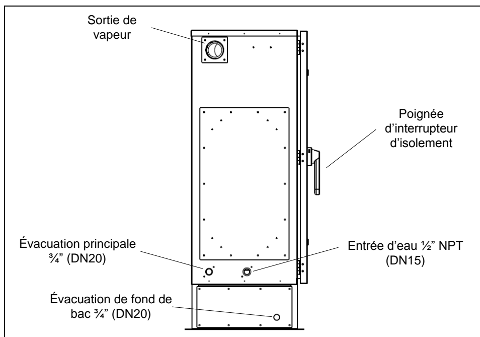
Illustration 40 - Raccordement de plomberie pour boîtier extérieur : vue de côté
