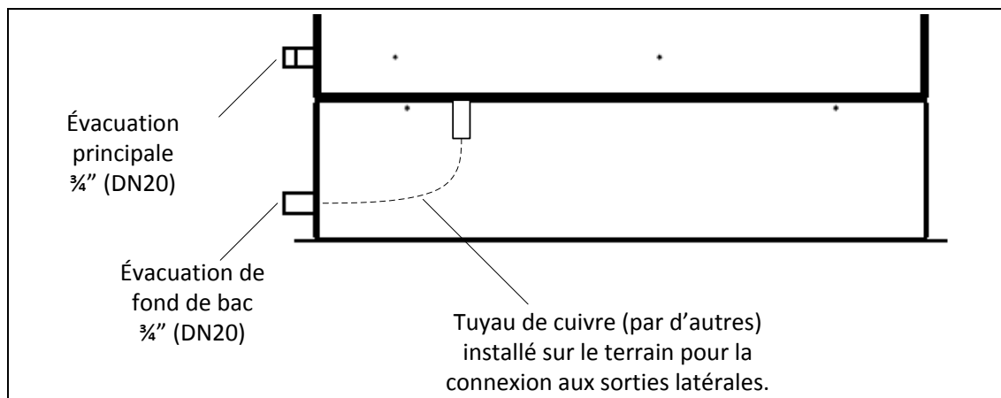
Illustration 39 - Raccordement de plomberie pour boîtier extérieur : vue frontale
