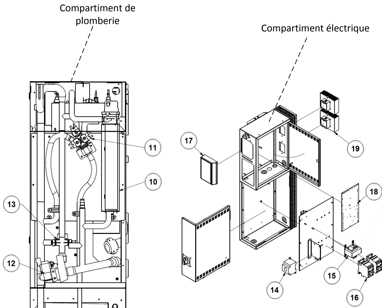
Illustration 56 - Vue explosée partie 2
