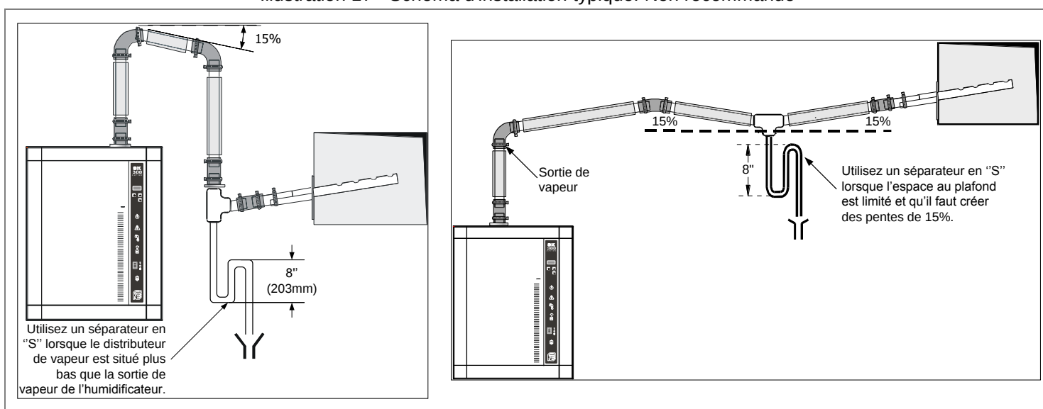
Illustration 18 - Séparateur de vapeur (S piège) installation
