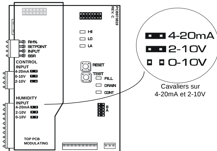
Illustration 32 - Signal 4 à 20 mA
