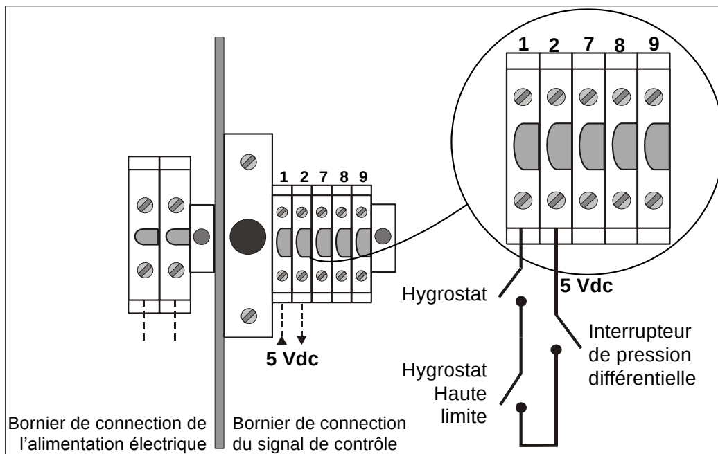
Illustration 26 - Connexions de contrôle basse tension
