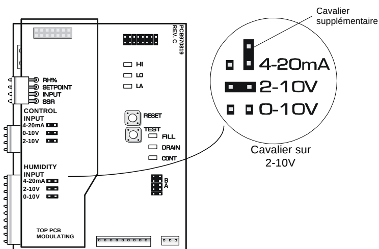
Illustration 31 - Signal 2 à 10 Vcc
