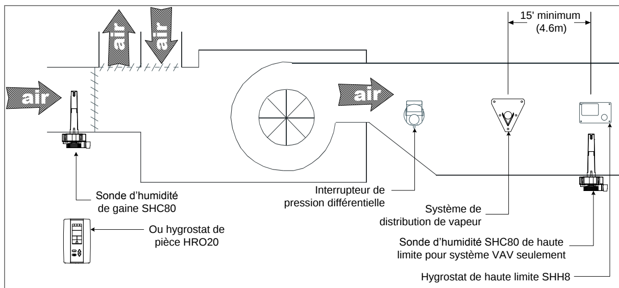
Illustration 37 - Commandes Placement (vapeur dispersée dans un conduit ou CTA)
