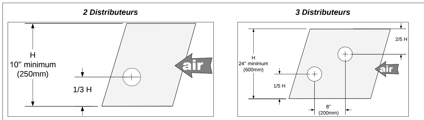
Illustration 12 - Distributeur 2 \frac{1}{8} " (54mm) diamètre emplacement: Conduits horizontaux
