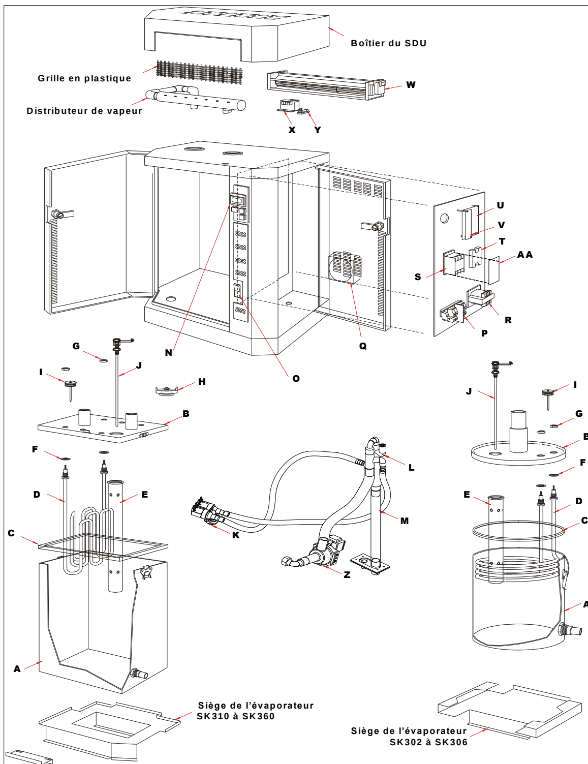
Illustration 43 - Vue explosée
