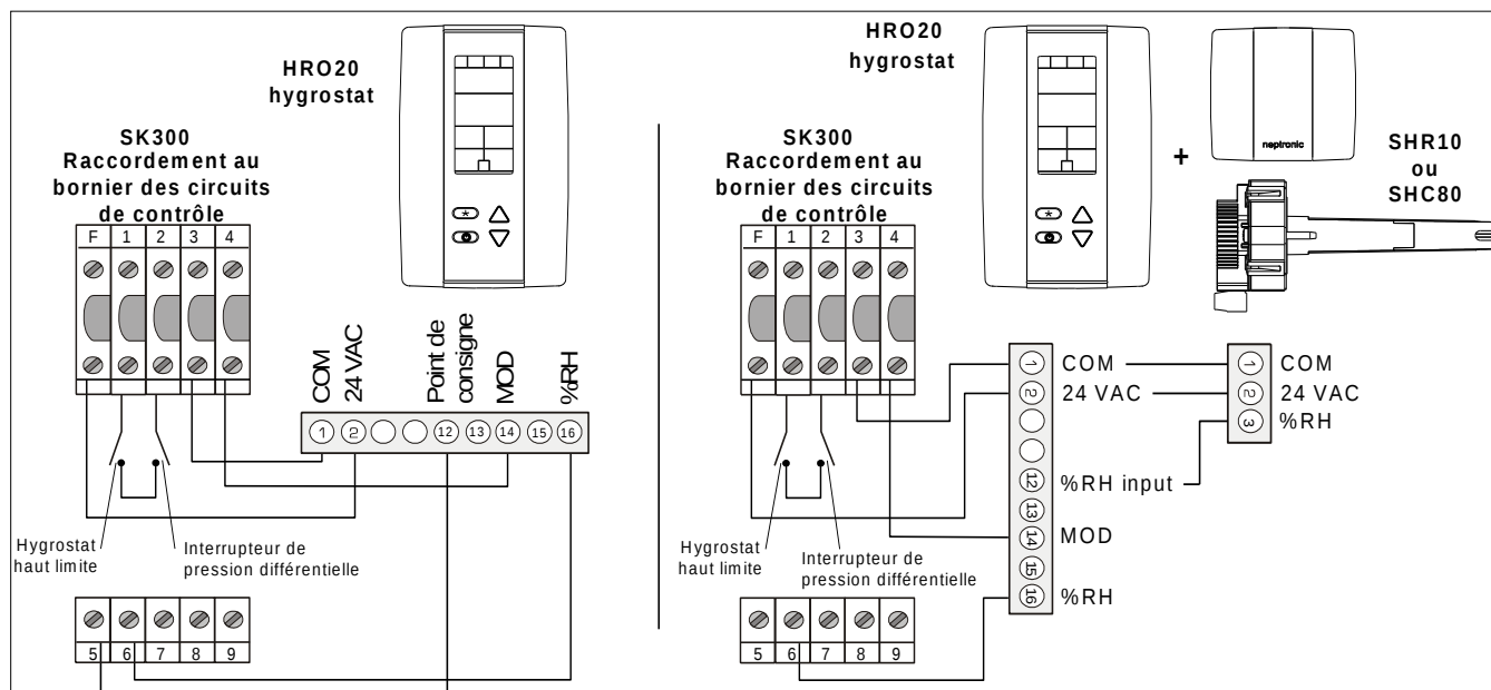
Illustration 27 - Connexion à HRO20 hygostat ou HRO20 avec capteur d'humidité à distance (SHR10 ou SHC80)
