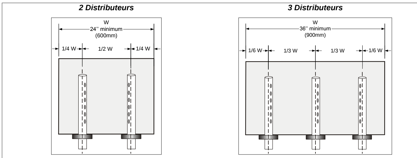
Illustration 15 - Distributeur 2 1/8" (54mm) diamètre emplacement: Conduits verticaux
