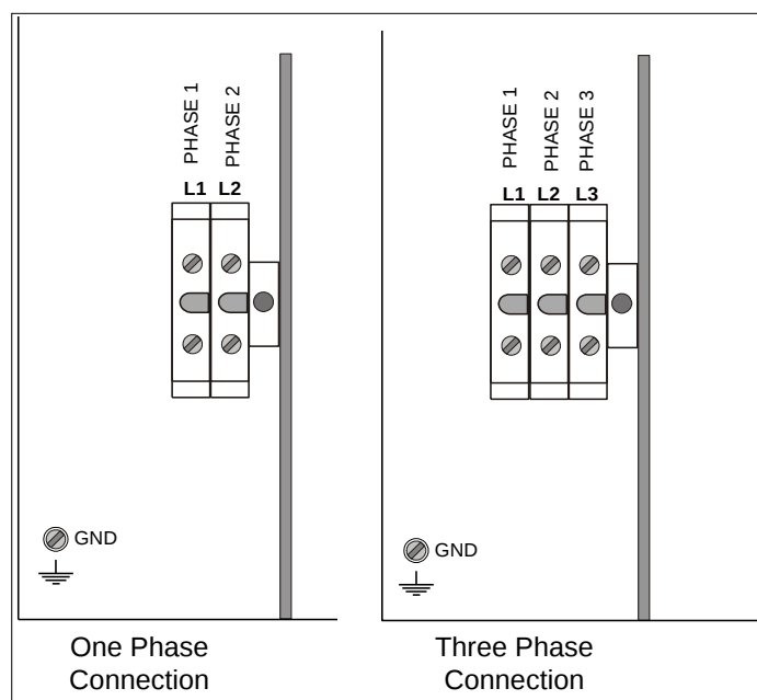
Illustration 25 - Raccordement électrique
