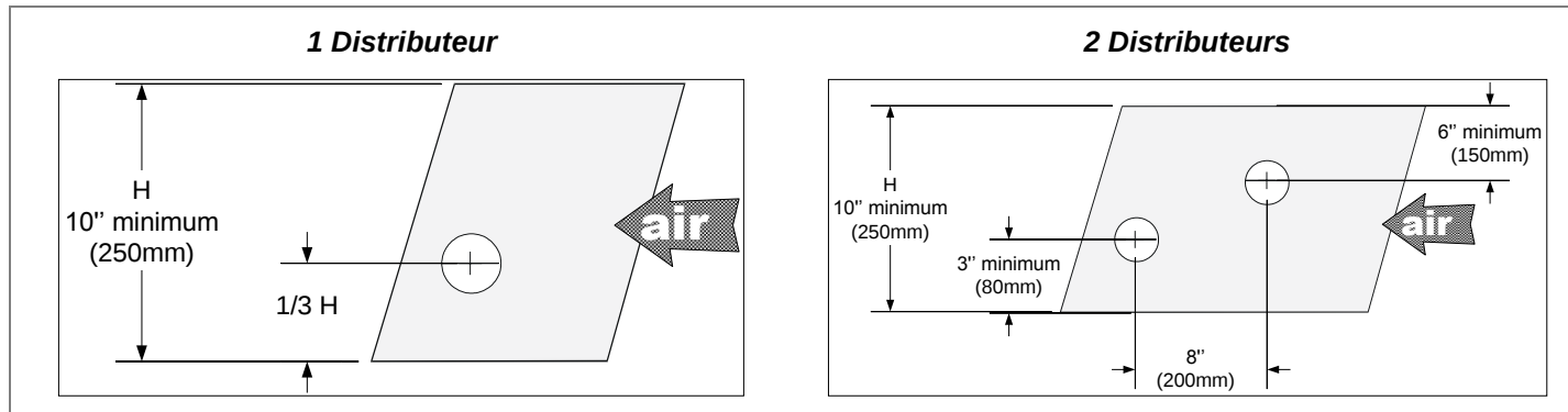
Illustration 11 - Distributeur 1 \frac{3}{8} " (35mm) diamètre emplacement: Conduits horizontaux
