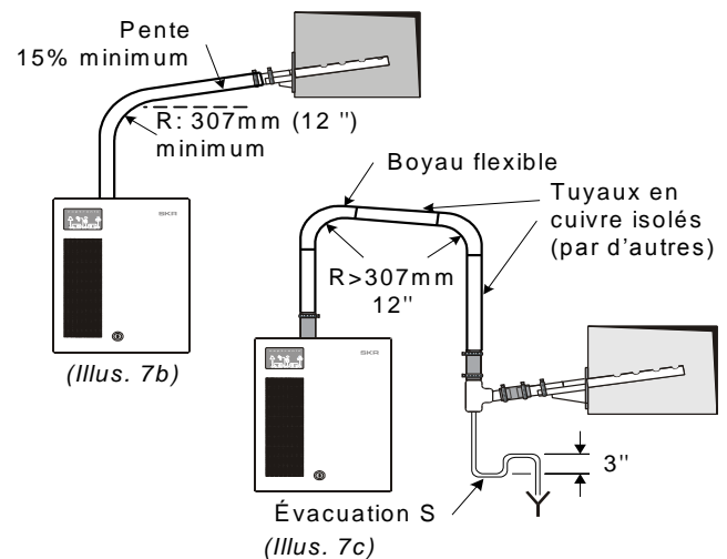
Installations recommandées
