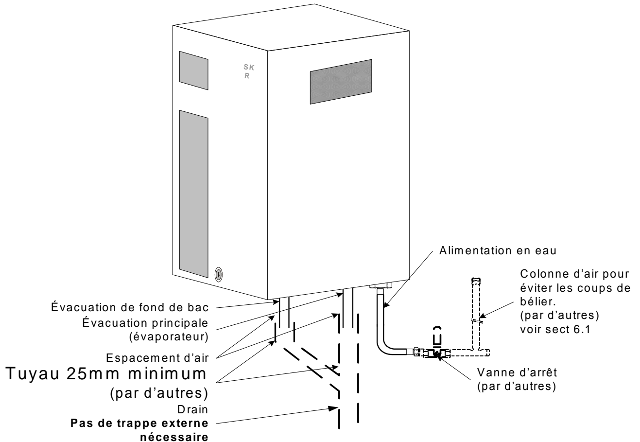
(Illus. 10a) Installation recommandée
